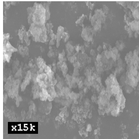
(Sol-gel)
